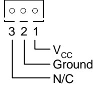
CN2 : ATX Control
